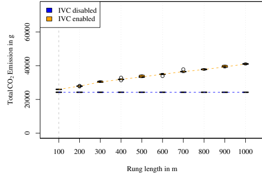
(d) ... influence on emissions
